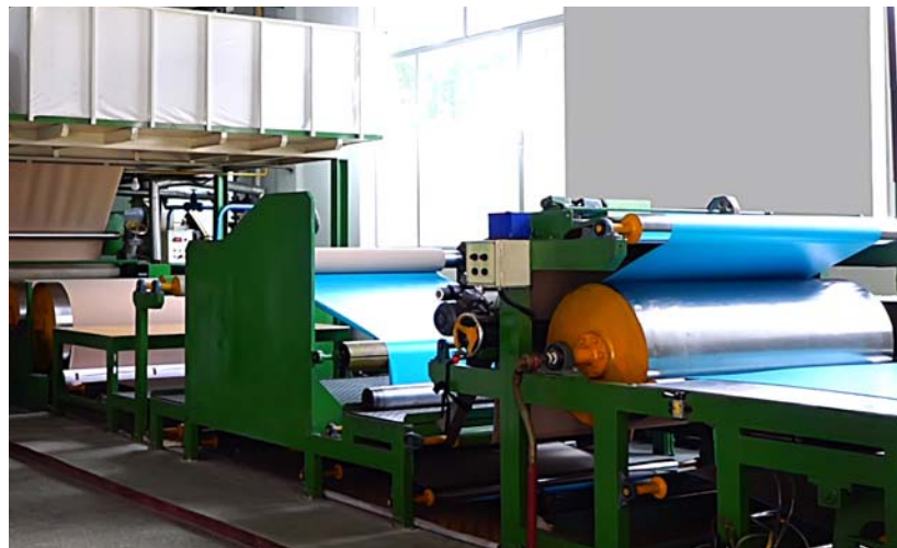
건식도포합성가죽생산공정
